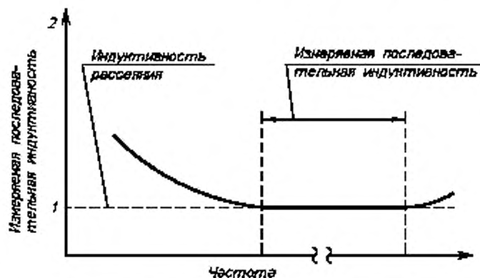
Рисунок 4 — Зависимость измеряемой последовательной индуктивности от частоты
