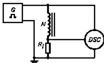
R_T — прецизионный резистор с чисто омическим сопротивлением вызывающий падение напряжения не превышающее 1 % от U_w
