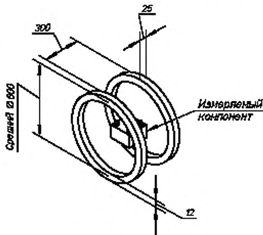
Рисунок 22 — Кольца Гельмгольца
