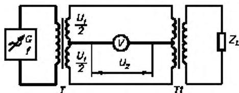
ТТ — испытываемый трансформатор
