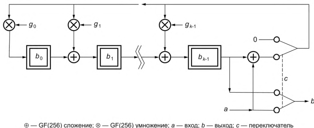
Рисунок 2 — Схема генерации кодовых слов исправления ошибки
