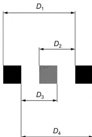
Рисунок 9 — Измерения расстояний от края до подобного края для определения центра каждого элемента
