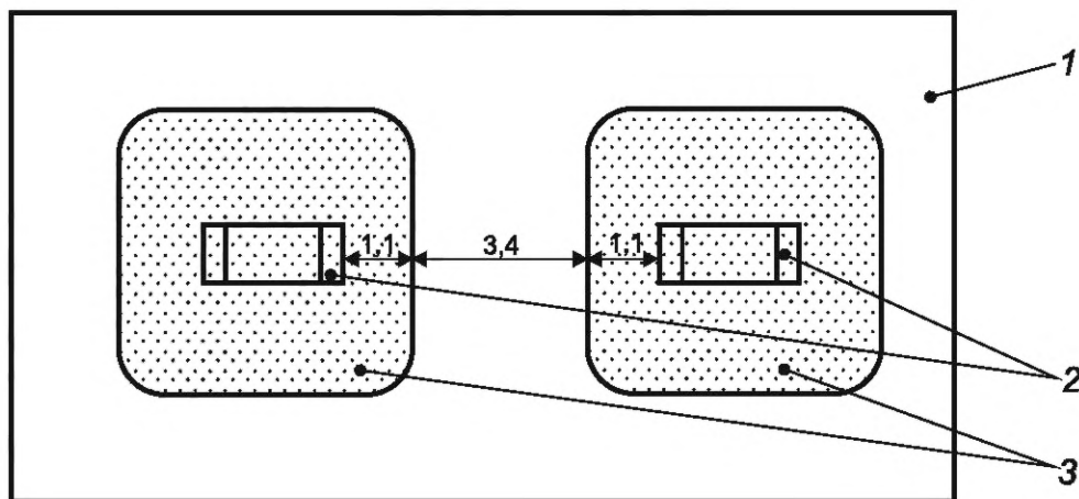
1 — печатная плата; 2 — электрический компонент; 3 — покрытие
