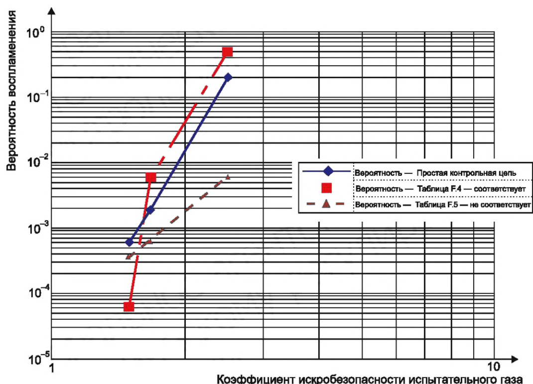
Рисунок F.1 — Зависимость вероятности воспламенения от коэффициента безопасности (коэффициент безопасности, обеспечиваемый взрывоопасными испытательными газовыми смесями)
