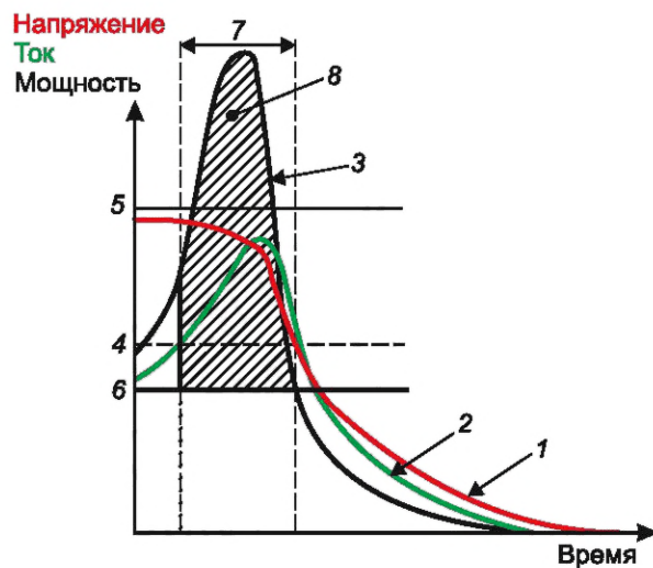
б) Пример превышения выходной энергии переходного процесса
