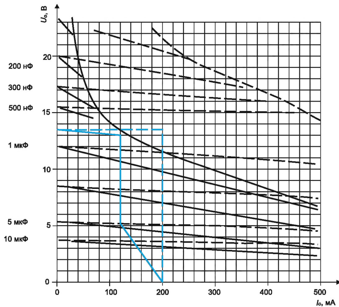
Рисунок G.1 — Примеры выходных характеристик для подгруппы IIS
