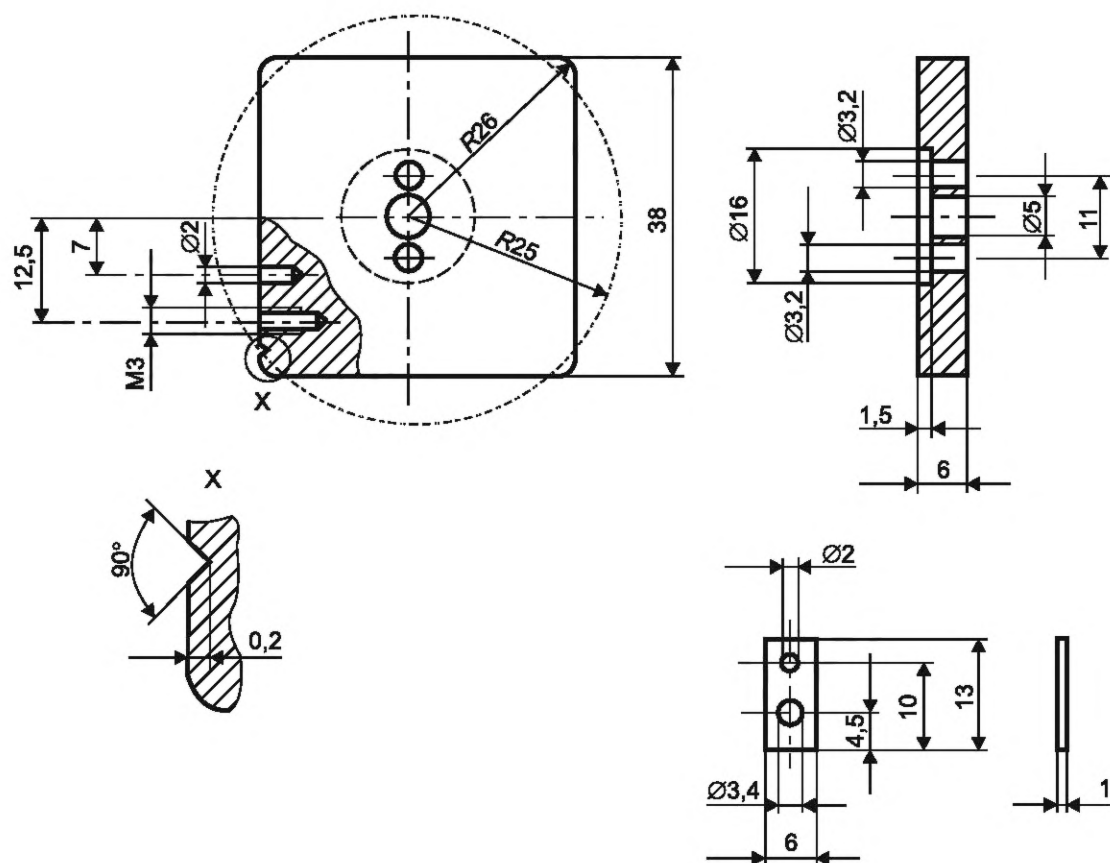
Рисунок В.3 — Держатель проволочек
