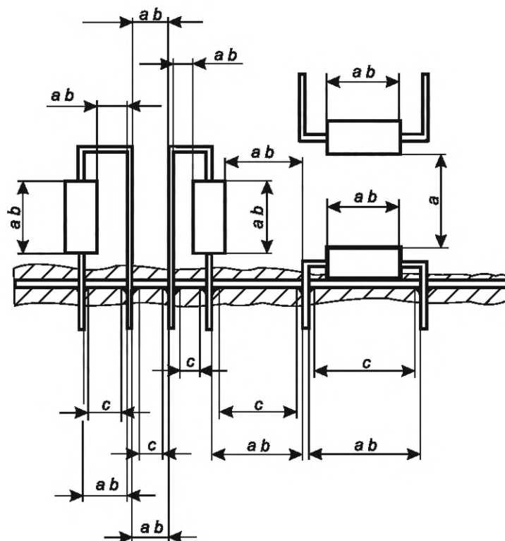
б) Сборка на печатной плате с выступающими из покрытия припаянными выводами
