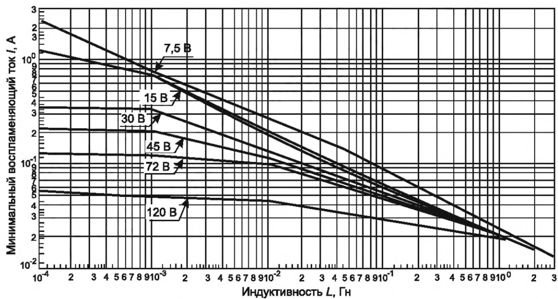
Рисунок А.4c — Индуктивные цепи подгруппы IIB
