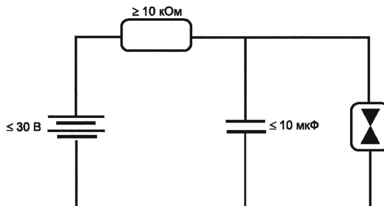
Рисунок 13 — Пример простой емкостной цепи
