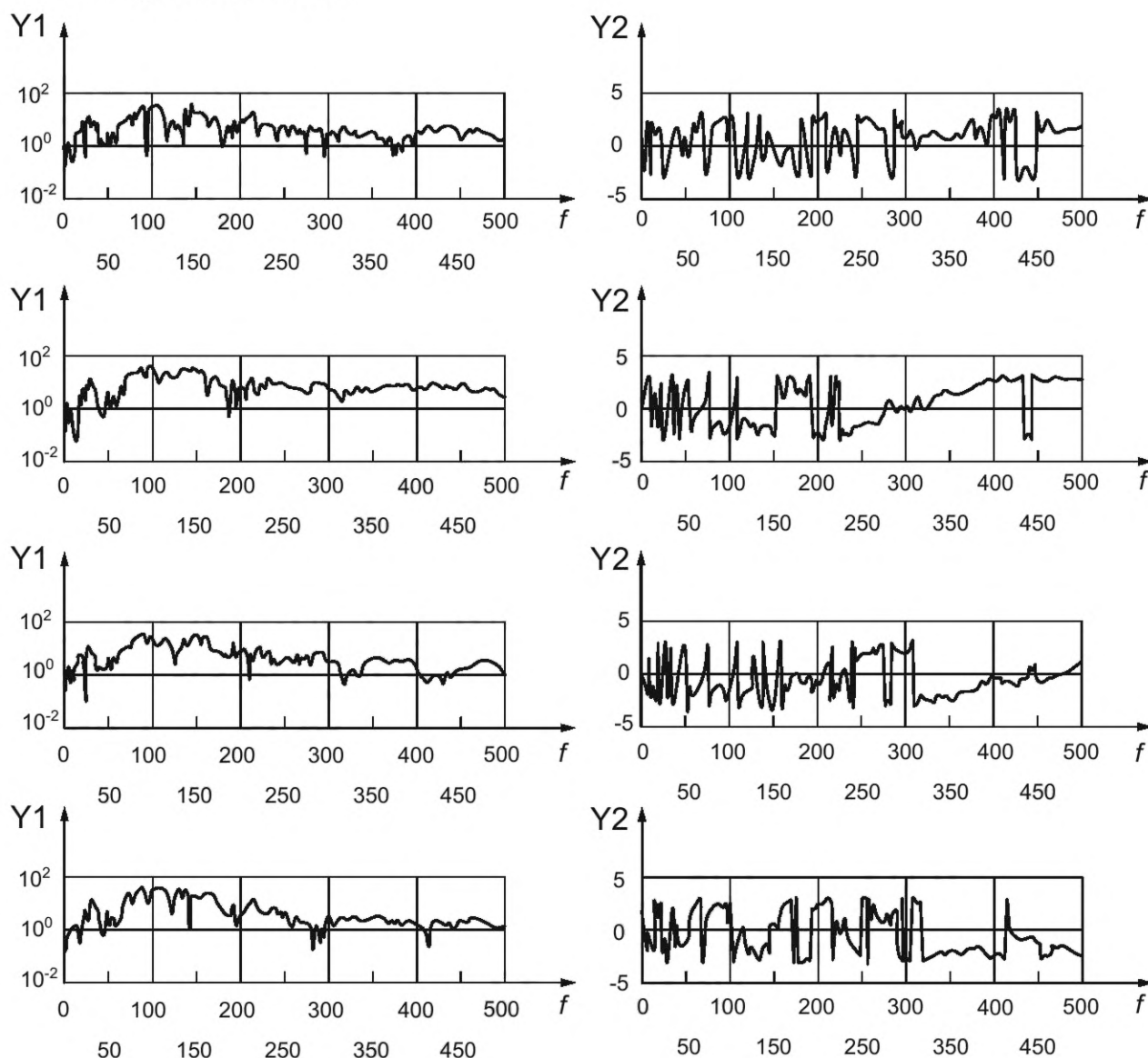
Рисунок А.5 — Графики амплитуды и фазы затормаживающих сил (сверху вниз) f_{b11} , f_{b12} , f_{b13} и f_{b14} (см. рисунки А.3 и А.4) с переменным разрешением по частоте
