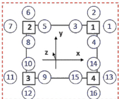
Рисунок С.4 — Иллюстративный материал к примеру 3 (квадратами с цифрами изображены упругие опоры, кружочками с цифрами — акселерометры в точках контроля)
