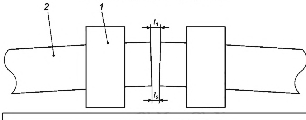
а) Имеются опорные ролики |l_1 - l_2| \leq 0,5 \text{ мм}
