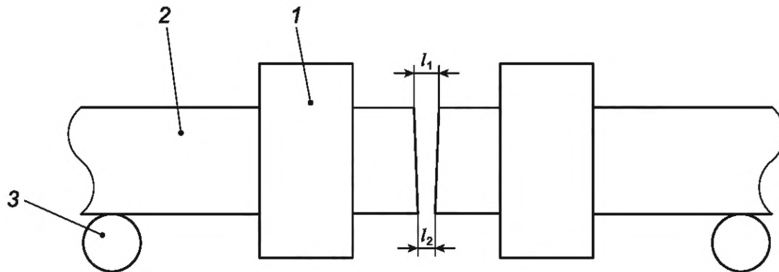
а) Имеются опорные ролики |l_1 - l_2| \leq 0,5 \text{ мм}
