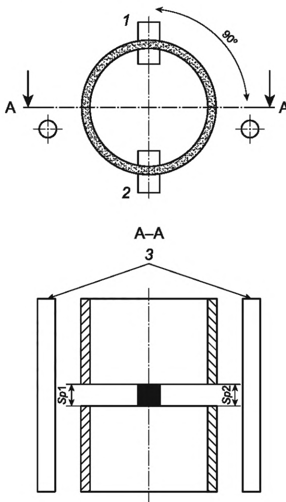
1, 2 — калиброванные блоки на осевой линии труб (со смещением на 90^\circ относительно направляющих элементов, например трубы, расположенной горизонтально с расположенными ниже направляющими элементами); 3 — направляющие элементы; Sp1 — размер в верхней точке; Sp2 — размер в нижней точке
