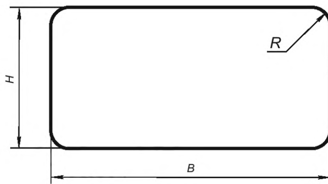
Рисунок 1 — Прессованный прямоугольный профиль полоsoобразного сечения
