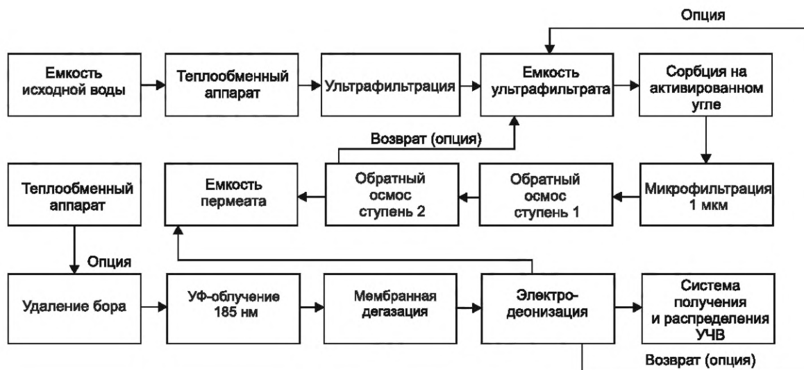
Рисунок В.1 — Блок-схема получения подпиточной (сверхчистой) воды в системе водоподготовки УЧВ (типы Е1.3, Е1.4)
