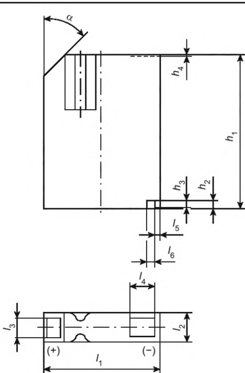
Рисунок 20 — Габаритный чертеж 4LR61
