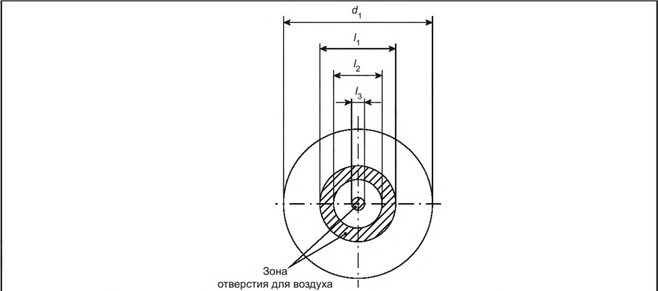
Рисунок 13 — Размещения отверстий подачи воздуха для батарей Р-системы
