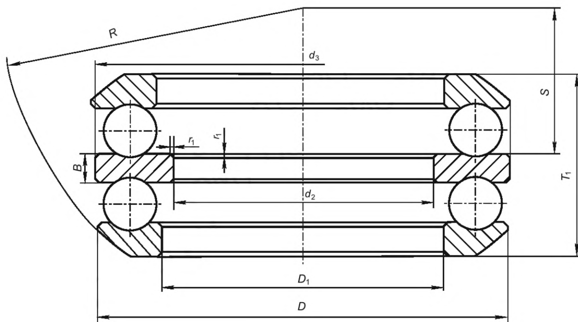
Рисунок 6 — Конструктивное исполнение 05
