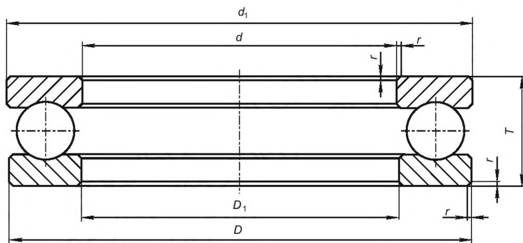
Рисунок 1 — Конструктивное исполнение 00
