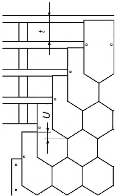
t — шаг обрешетки; U — расстояние от нижнего края перекрывающей плитки до верхней кромки плитки предыдущего перед перекрываемым ряда
