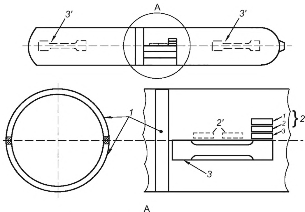
1 — расположение места отбора образцов на изгиб или образца в виде кольца для сплющивания; 2 — расположение места отбора продольных образцов для испытания на ударный изгиб (с условными номерами образцов); 2' — альтернативное расположение места отбора продольных образцов для испытания на ударный изгиб; 3 — расположение места отбора образца для испытания на растяжение; 3' — альтернативное расположение места отбора образца для испытания на растяжение
