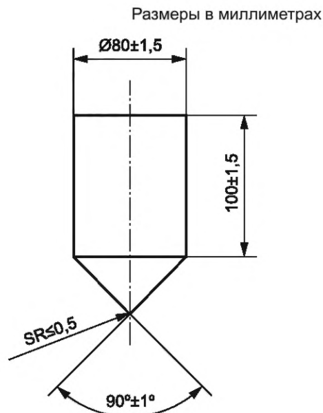
Рисунок 6 — Испытательный конус
