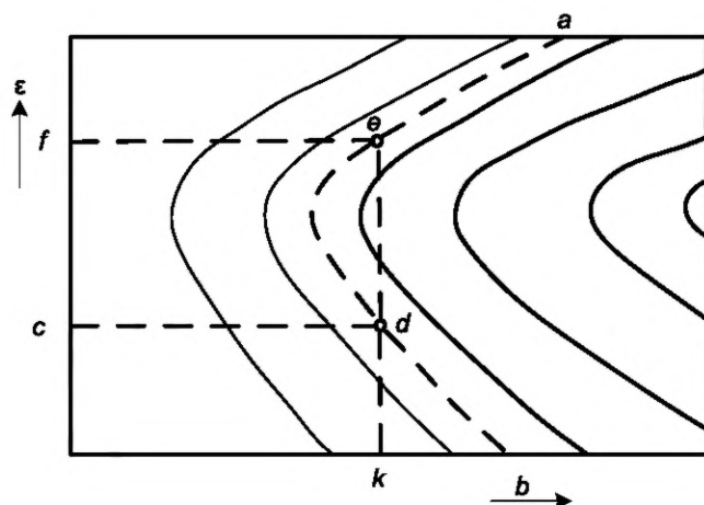
Рисунок 4 — Схема графика для определения взаимных глубин в гидравлическом прыжке при трапецеидальном русле
