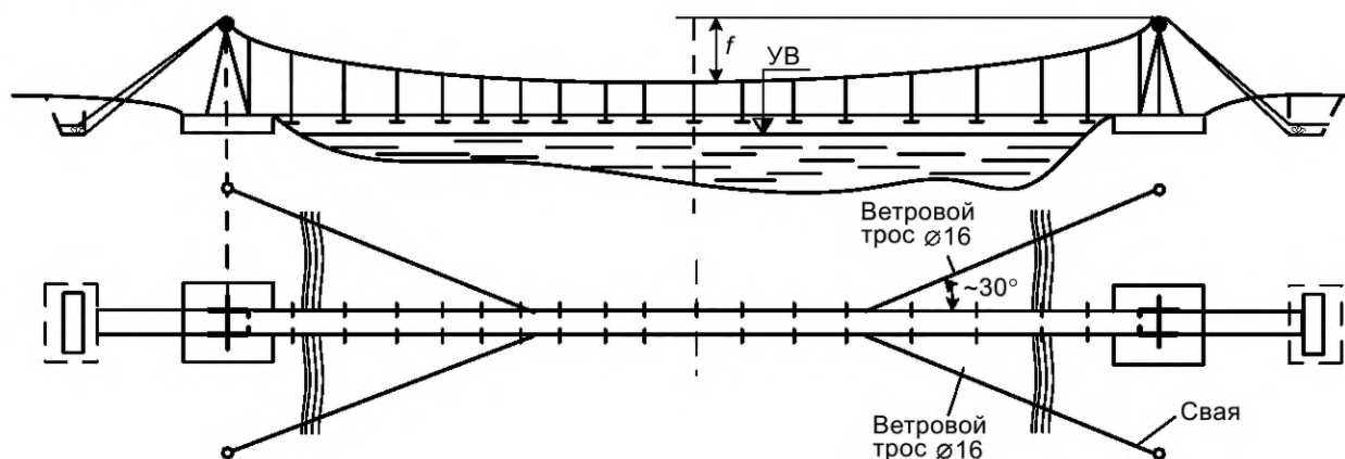
Рисунок В.4 — Продольный разрез и план подвесного гидрометрического мостика
