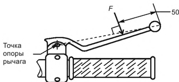
Рисунок 2 — Расположение точки приложения усилия к рычагу управления
