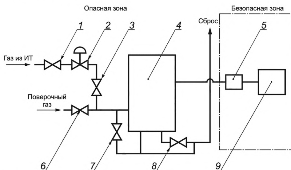
1 — изолирующий клапан; 2 — регулятор давления; 3, 6, 7, 8 — клапаны; 4 — плотномер; 5 — барьер искрозащиты; 9 — вычислитель Рисунок 7 — Типовая схема монтажа потокового плотнмера для измерения плотности газа при стандартных условиях
