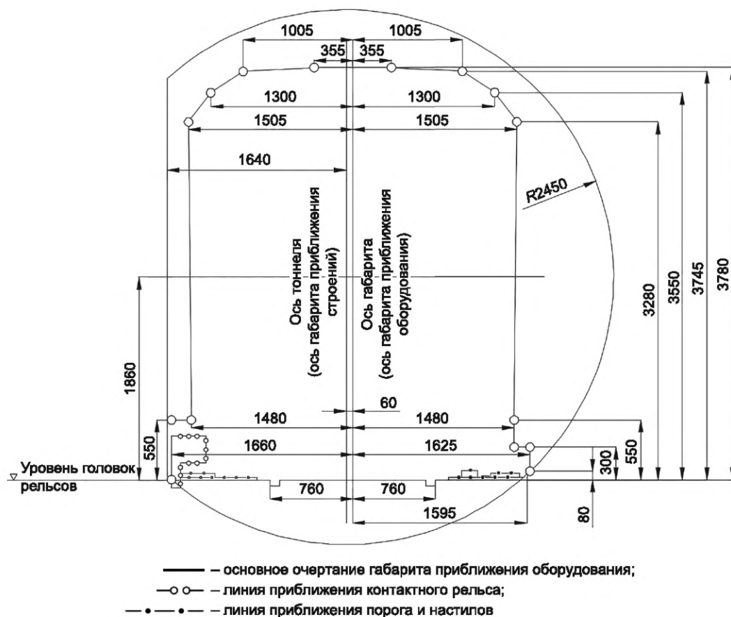
Рисунок 15 — Совмещенные габариты приближения строений C_{м3} и приближения оборудования O_{м3} для станций закрытого типа
