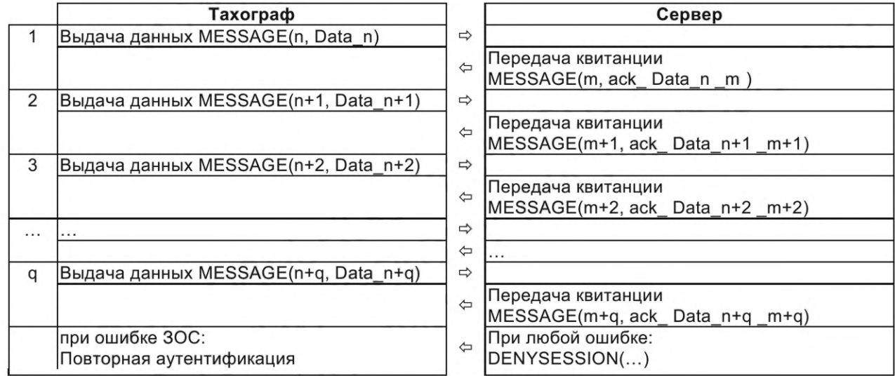
Рисунок 2 — Схема обмена сообщениями тахографа и сервера
