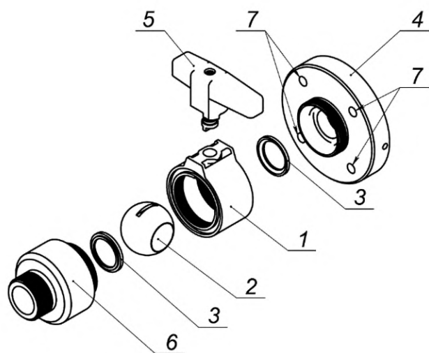
Рисунок 1 — Конструктивные элементы КШ
