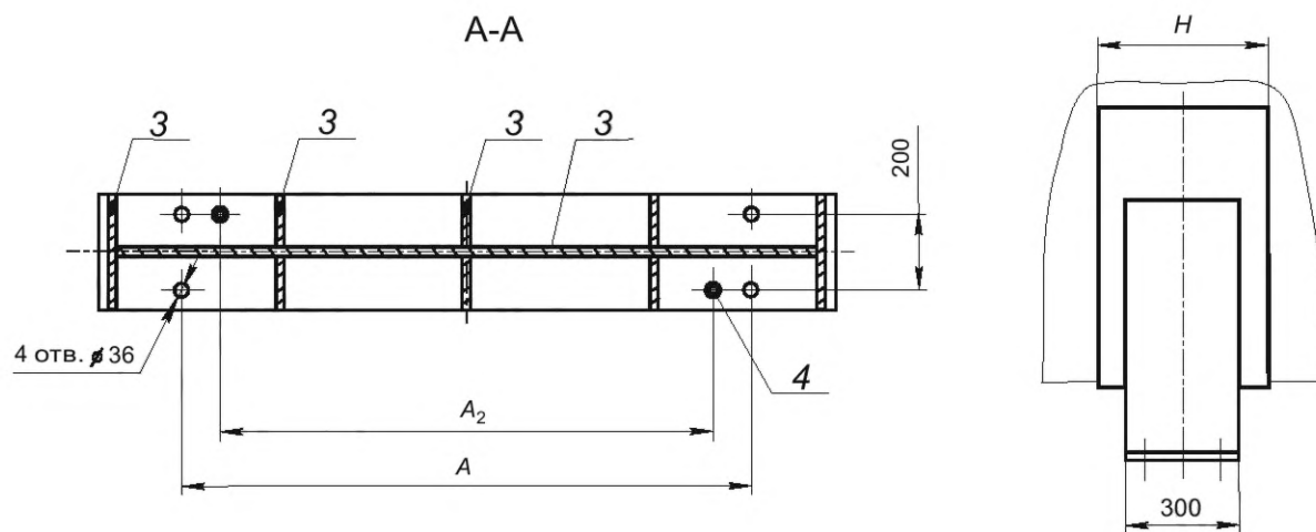
Рисунок 6 — Конструкция неподвижной опоры типа 3
