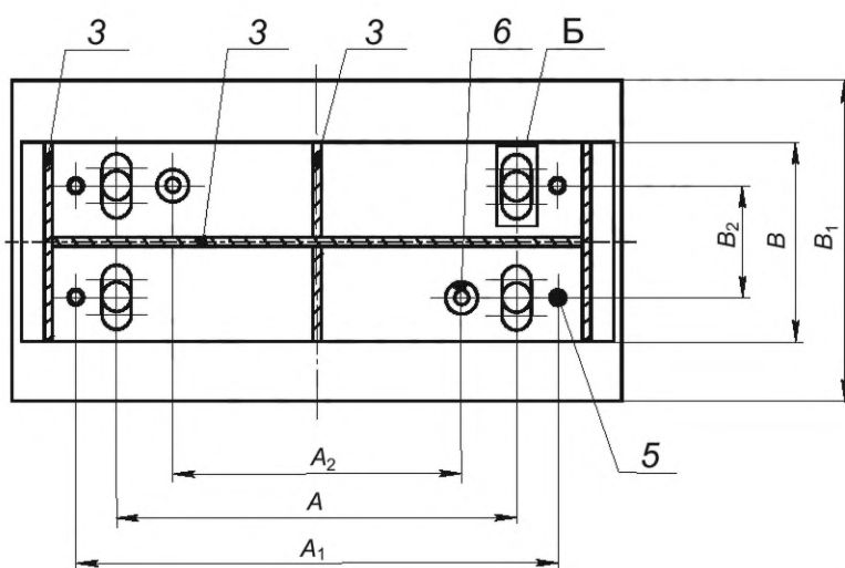
Рисунок 3 — Конструкция подвижной опоры типа 2
