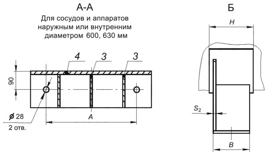
1 — опорный лист; 2 — опорная плита; 3 — ребро; 4 — ребро
