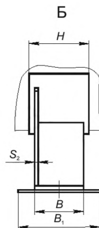
Рисунок 1 — Конструкция подвижной опоры типа 1
