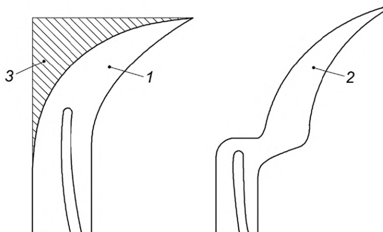
1 — пример приемлемой формы раскливающего ножа; 2 — пример неприемлемой формы раскливающего ножа; 3 — заштрихованная область: зона раскливающего ножа для установки в ней защитного кожуха дисковой пилы
