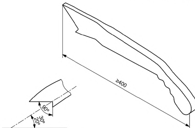
Рисунок 16 — Пример палочного толкателя
