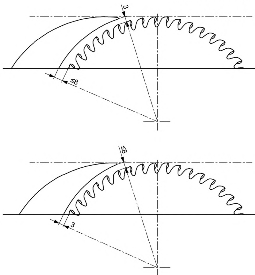
Рисунок 10 — Предельные значения позиционирования раскливающего ножа
