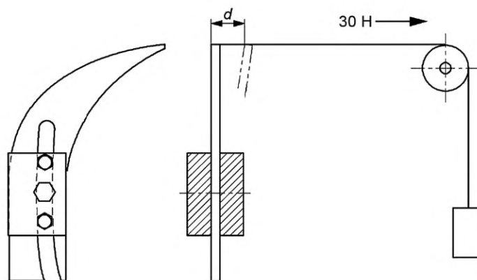
Рисунок I.2 — Проверка поперечной жесткости расклинивающего ножа
