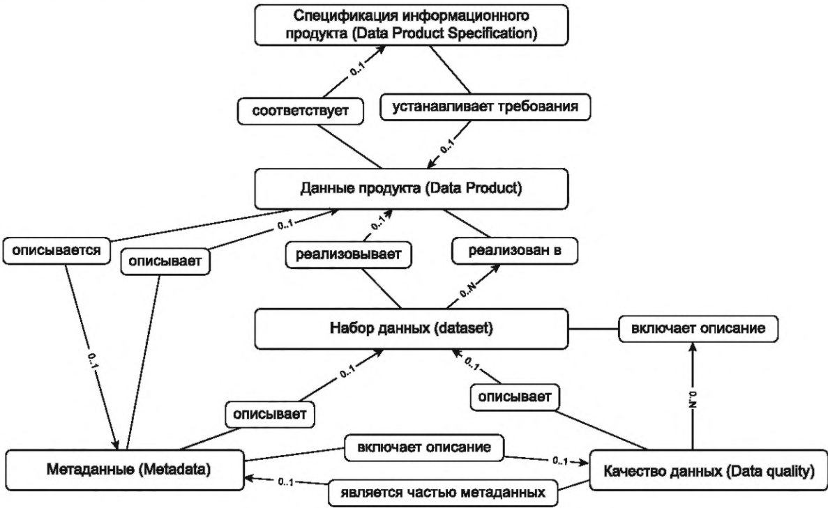
Рисунок Б.1 — Взаимодействие спецификации, данных и метаданных
