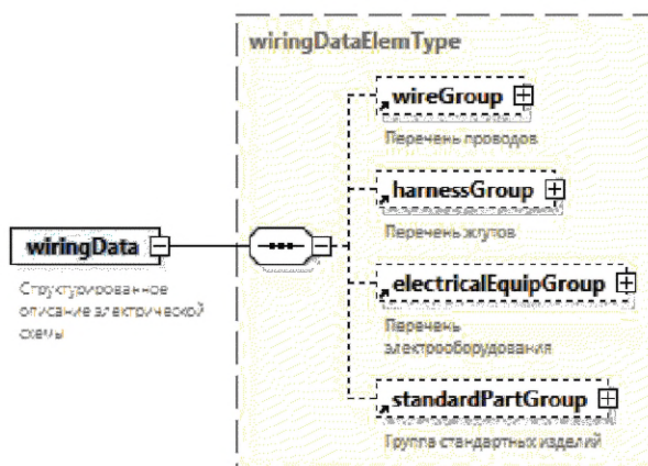
Рисунок A.35 — Схема элемента <wiringData>
