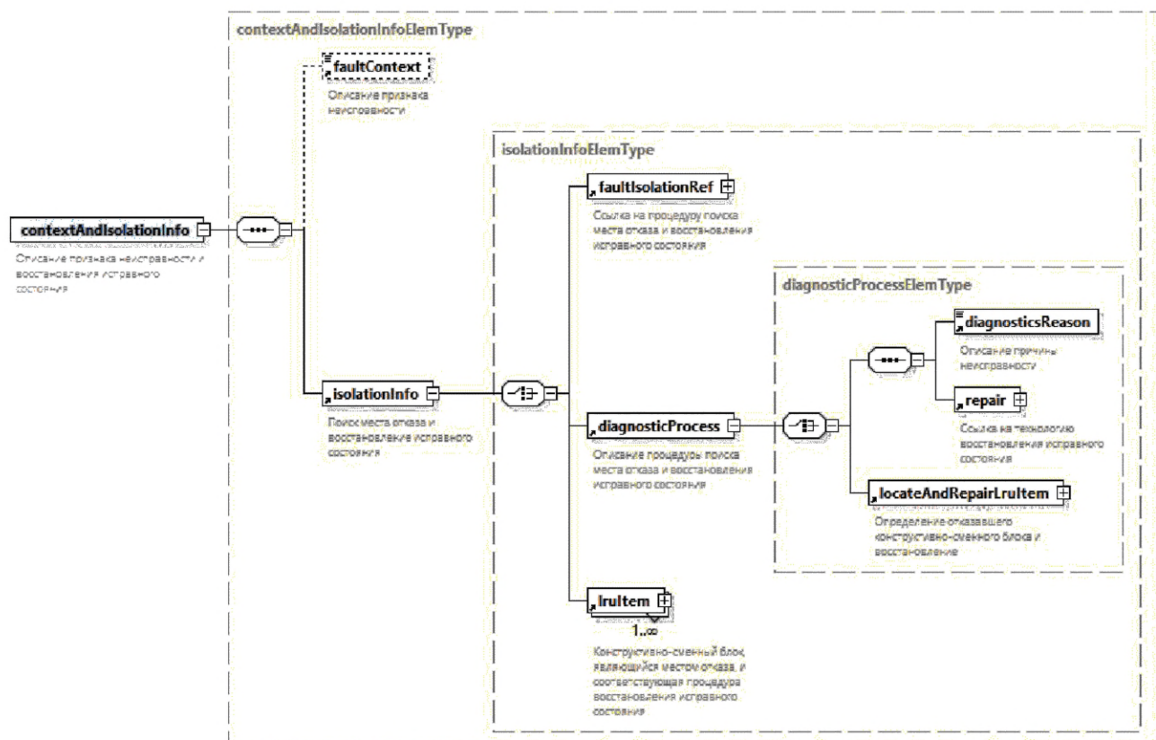
Рисунок А.30 — Схема элемента &lt;contextAndIsolationInfo&gt;
