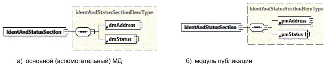
Рисунок А.2 — Верхнеуровневая структура РЧ МД
