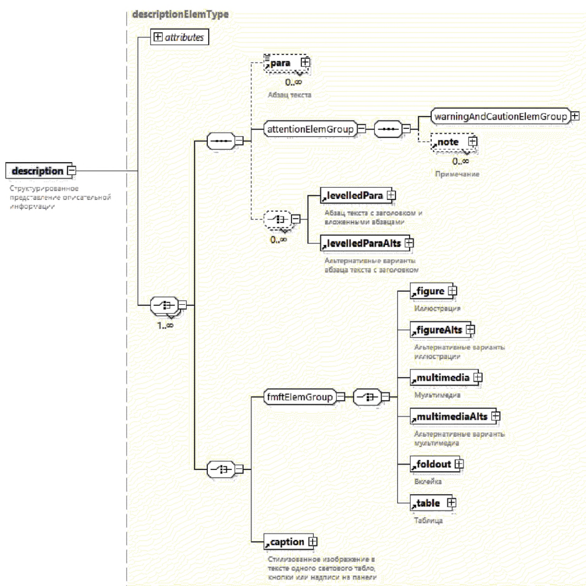
Рисунок А.19 — Схема элемента <description>
