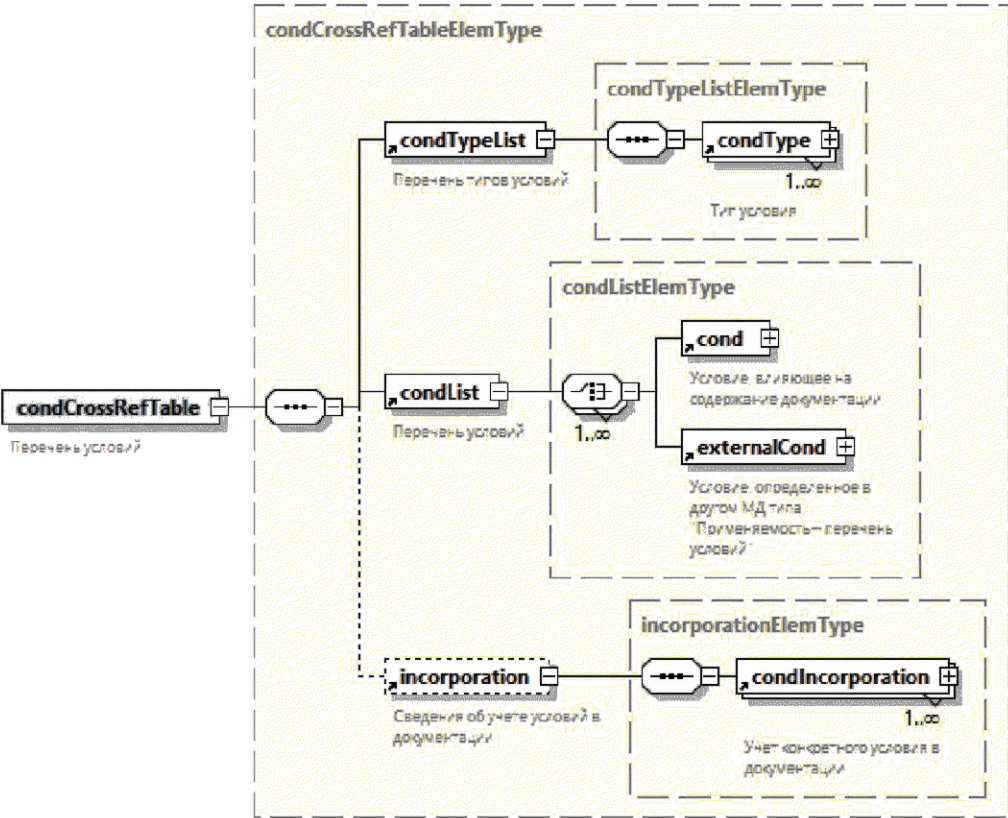
Рисунок А.40 — Схема элемента <condCrossRefTable>
