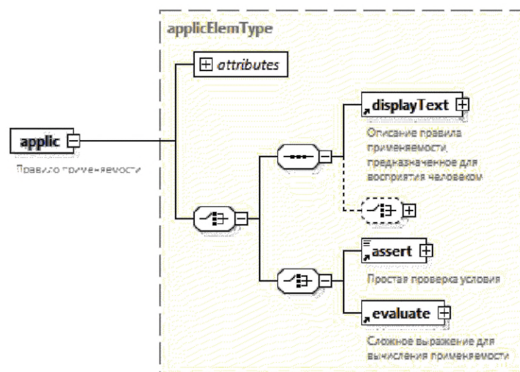
Рисунок А.15 — Схема элемента &lt;applic&gt;
