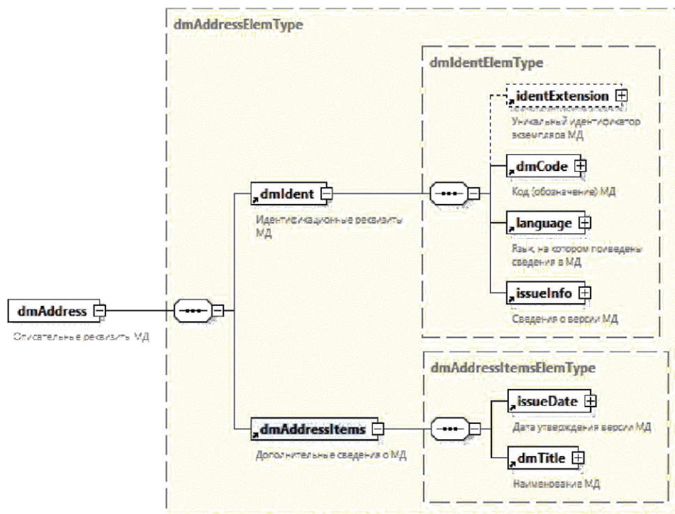
Рисунок А.3 — Структура описательных реквизитов основного (вспомогательного) МД
