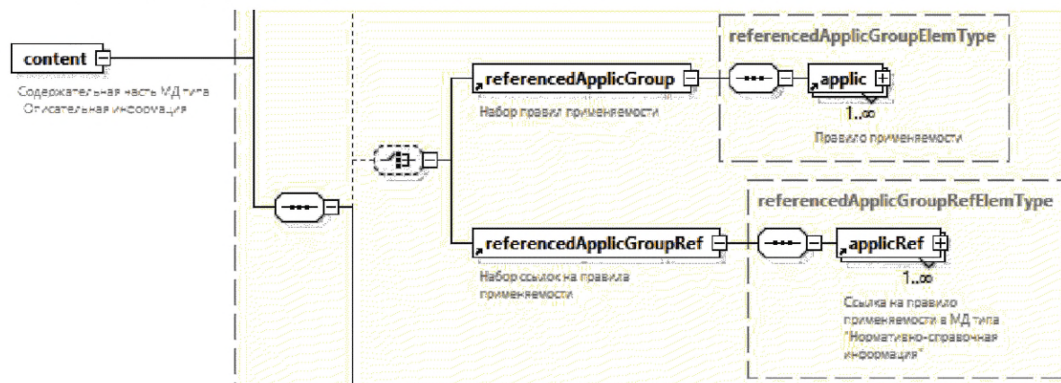
Рисунок А.16 — Представление правил применимости для содержимого МД в элементе &lt;content&gt;
