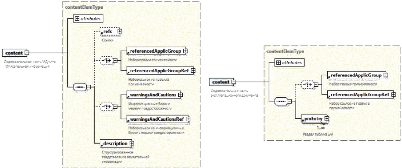
а) основной и вспомогательный МД (пример для МД типа «Описательная информация»)
