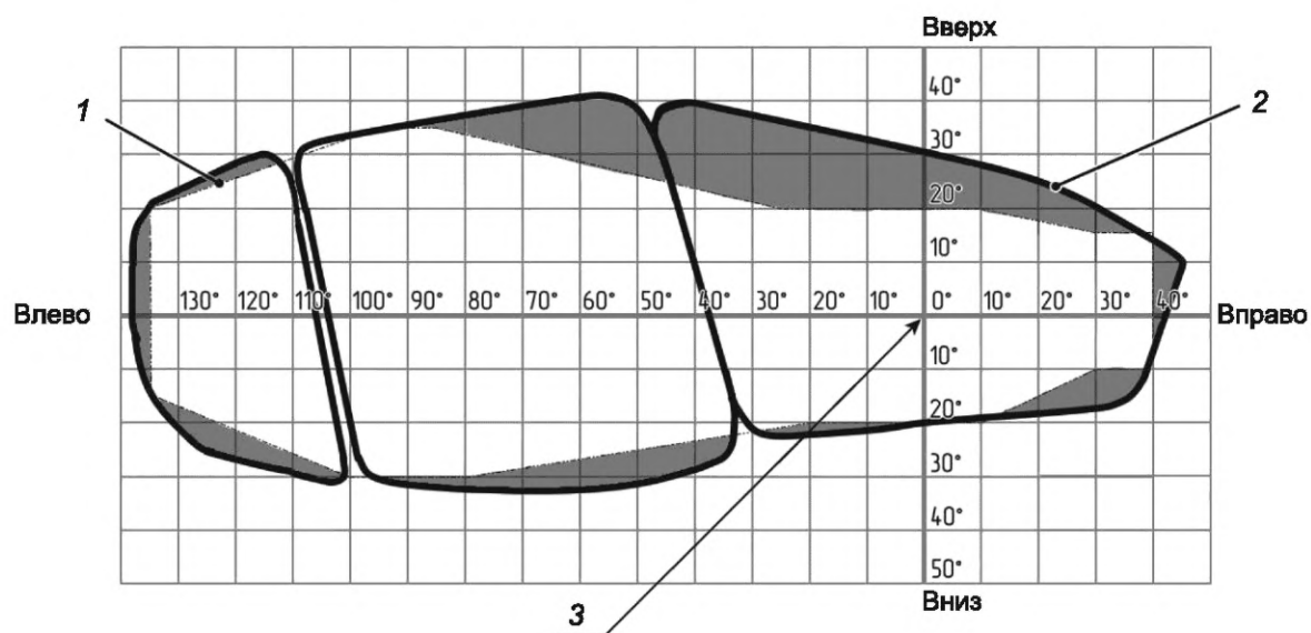
Рисунок Б.1 — Пример построения диаграммы обзора из двухместной кабины самолета для летчика, расположенного в кабине слева
