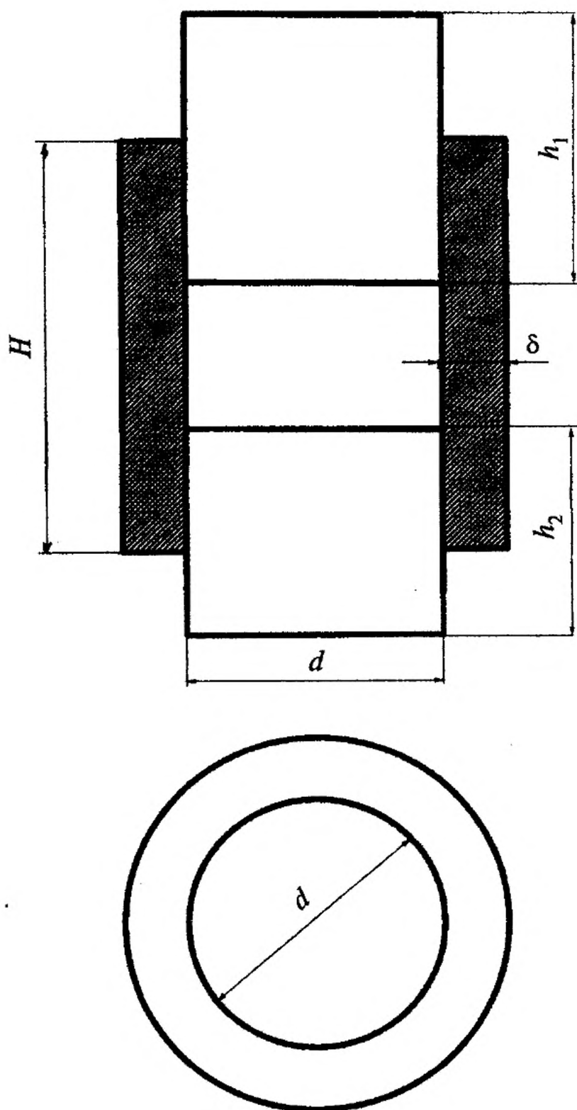
Рисунок 2 — Форма для изготовления образцов
