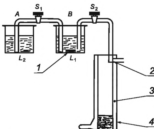
А — сосуд с менее плотной жидкостью L_2 ; В — сосуд с более плотной жидкостью L_1 ; S_1 — сифон сосуда А; S_2 — сифон сосуда В; 1 — магнитная мешалка; 2 — термостат; 3 — капилляр, касающийся внутренней поверхности колонки; 4 — колонка
