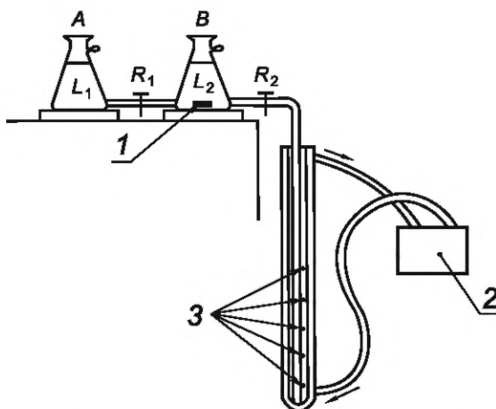
А — сосуд с более плотной жидкостью L_1 ; В — сосуд с менее плотной жидкостью L_2 ; R_1 — кран сосуда А; R_2 — кран сосуда В; 1 — магнитная мешалка; 2 — водяная оболочка с термостатическим регулированием; 3 — эталонные поплавки
