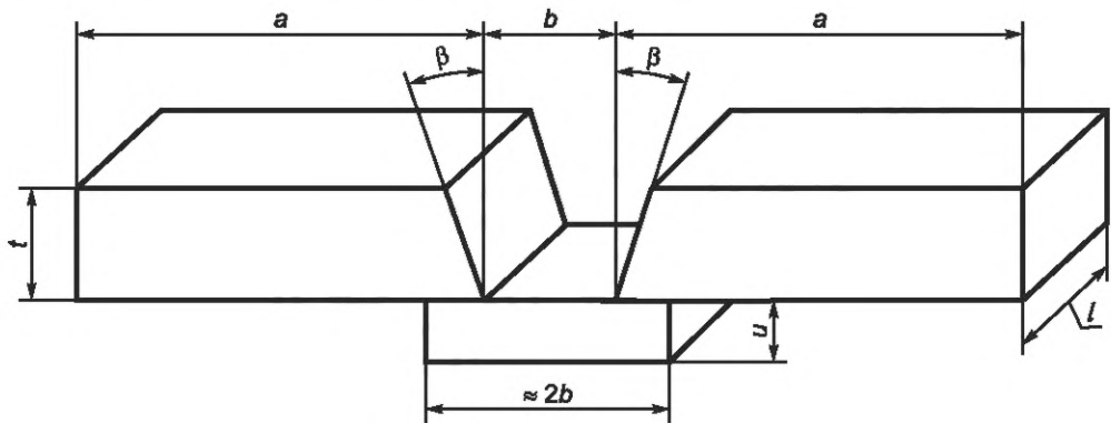
Рисунок 1 — Размеры заготовки
