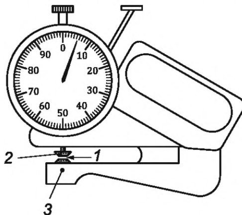
1 — наковальня; 2 — верхний измерительный наконечник; 3 — пята
