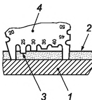
Рисунок 1 — Пример толщиномера-гребенки
