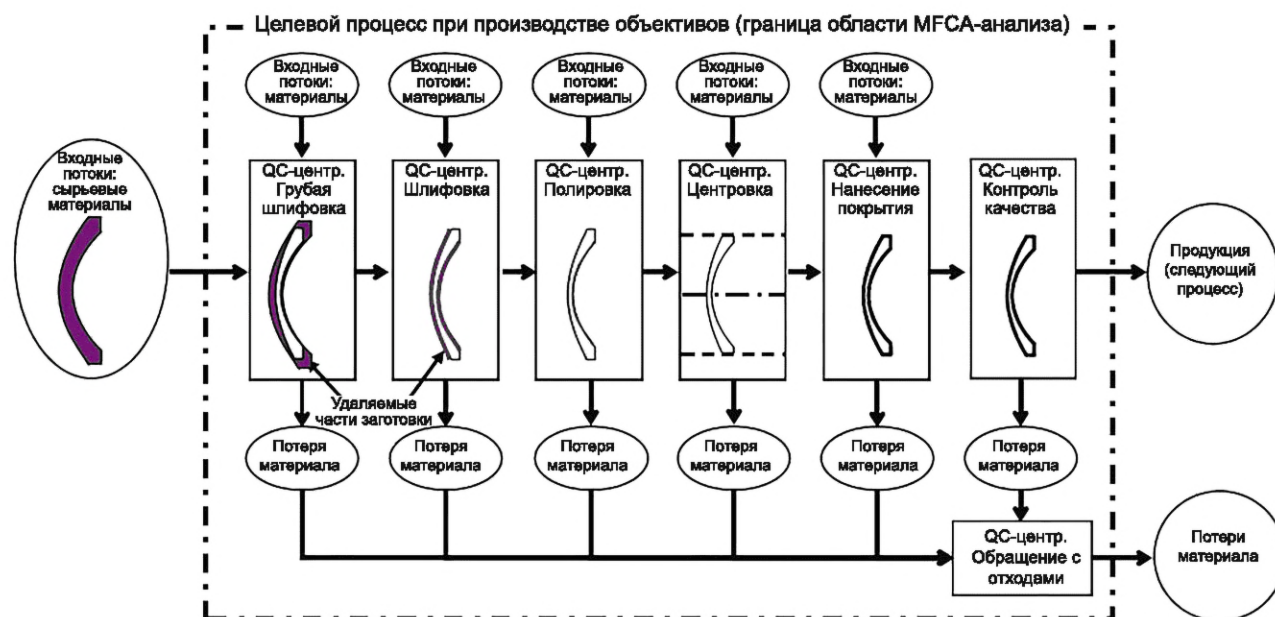
Рисунок С.1 — Модель потоков материалов в основном целевом процессе
