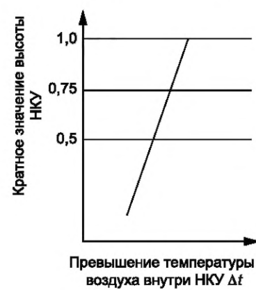
Рисунок F.5 — Пример 2, расчет для НКУ для настенного монтажа с вентиляционными отверстиями
