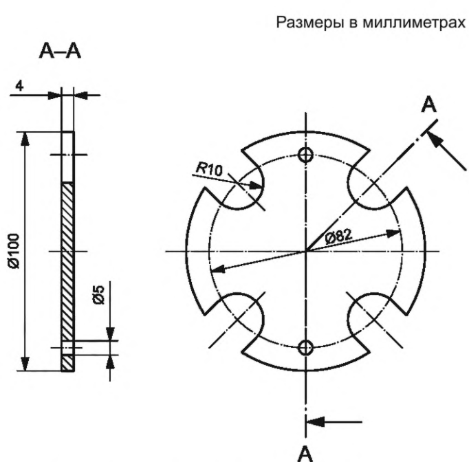
Рисунок 6 — Прозрачная крышка (необязательный компонент)
