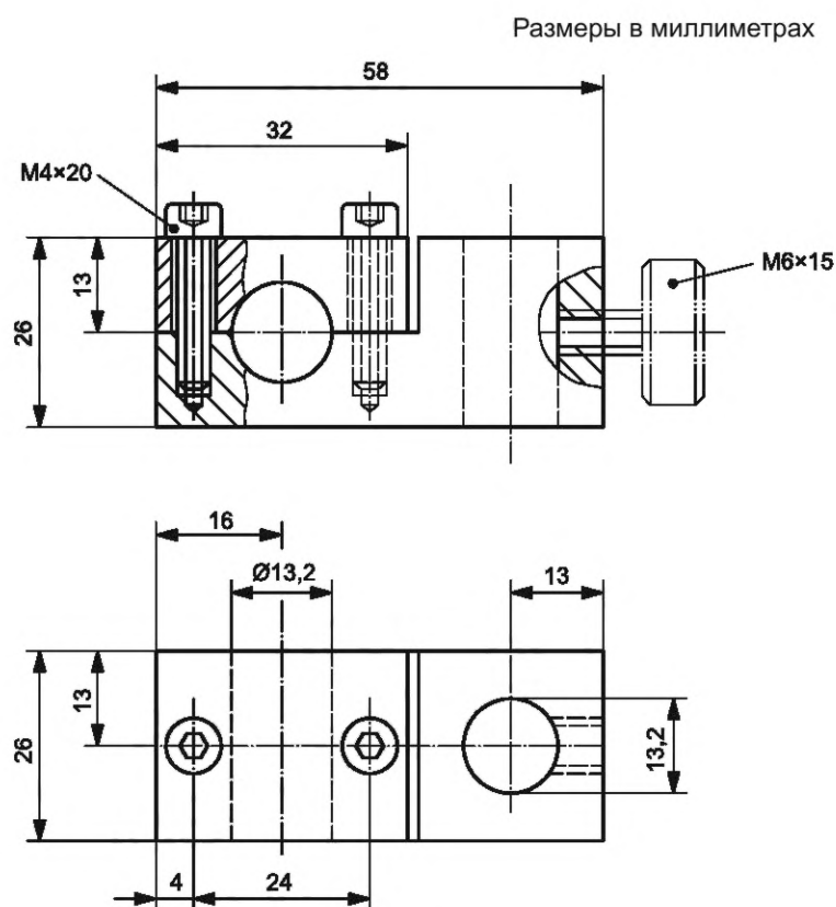
Рисунок 8 — Поворотный зажим
