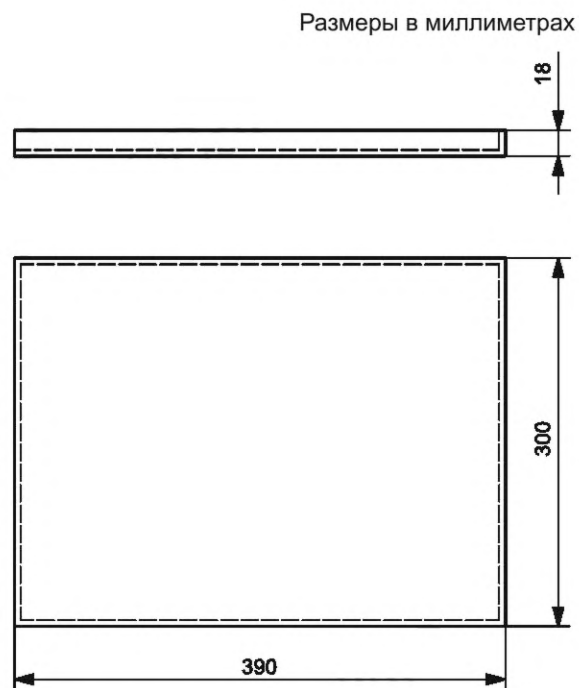
Рисунок 7 — Поддон
