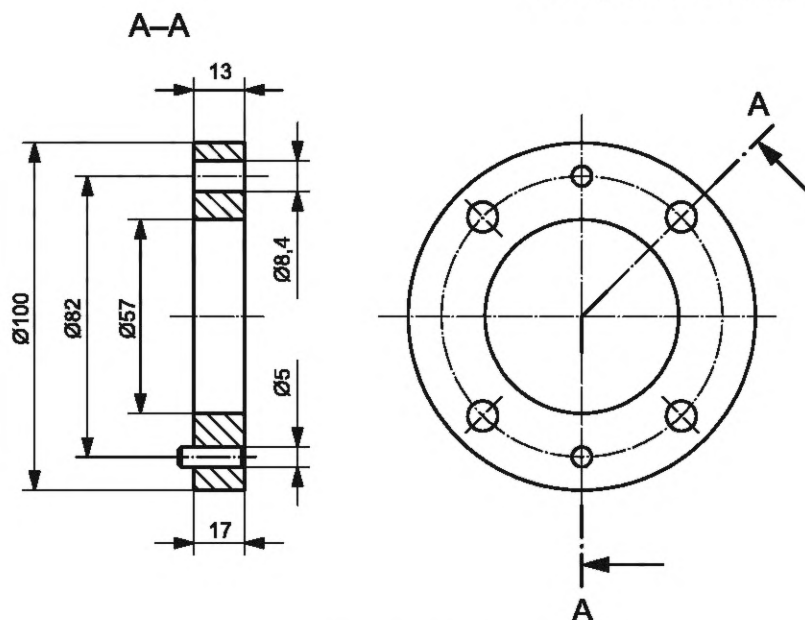
Рисунок 5 — Фланец
