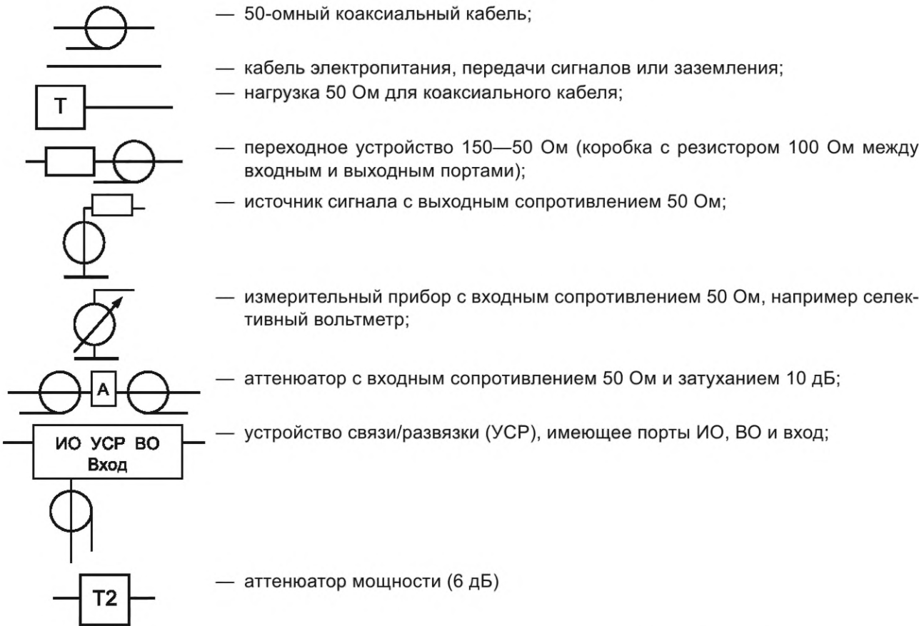
а) Перечень символов, применяемых для показа принципов ввода помехи и связи в схемах расположения оборудования при проведении испытания
