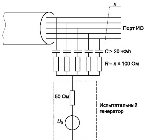
с) Принцип связи для неэкранированных кабелей в соответствии с методом применения УСР
