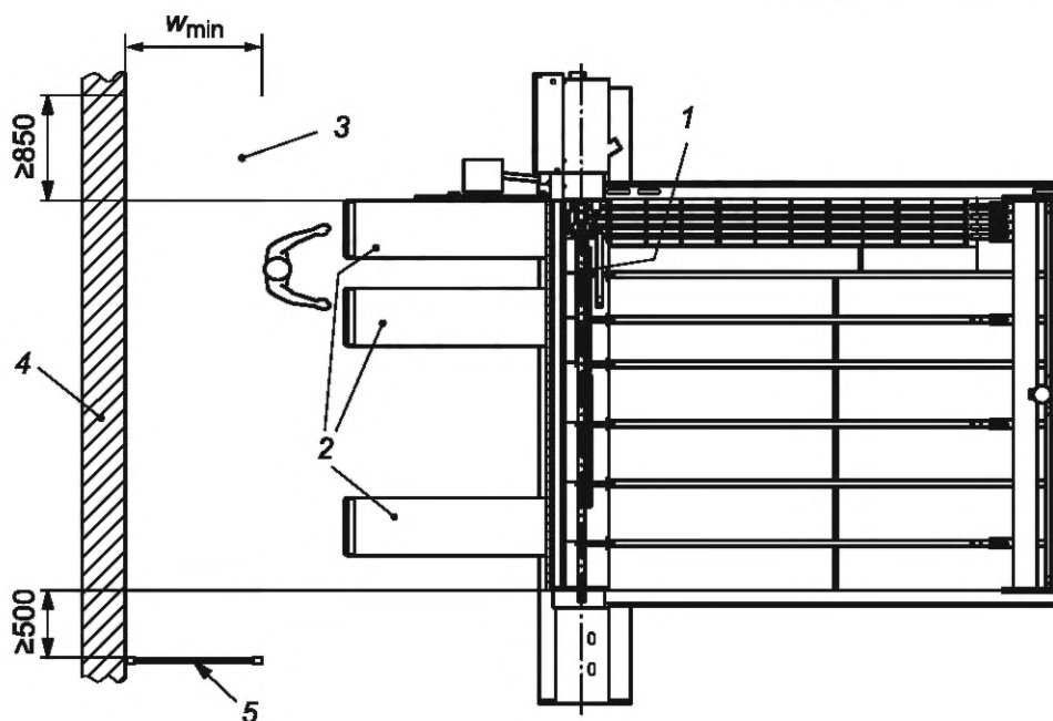
1 — передняя линия резания; 2 — удлинительные столы; 3 — ESPE или чувствительные к давлению маты; 4 — стена; 5 — ограждение; w_{\min} — минимальная ширина просвета
