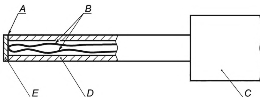
A — клей; B — провода термопары диаметром 0,3 мм по IEC 60584-1, тип К (хром-алюмель); C — расположение рукоятки, обеспечивающее усилие контакта (4 \pm 1) Н; D — поликарбонатная трубка: внутренний диаметр 3 мм, наружный диаметр 5 мм; E — диск из луженой меди: диаметр 5 мм, толщина 0,5 мм с плоской контактной поверхностью
