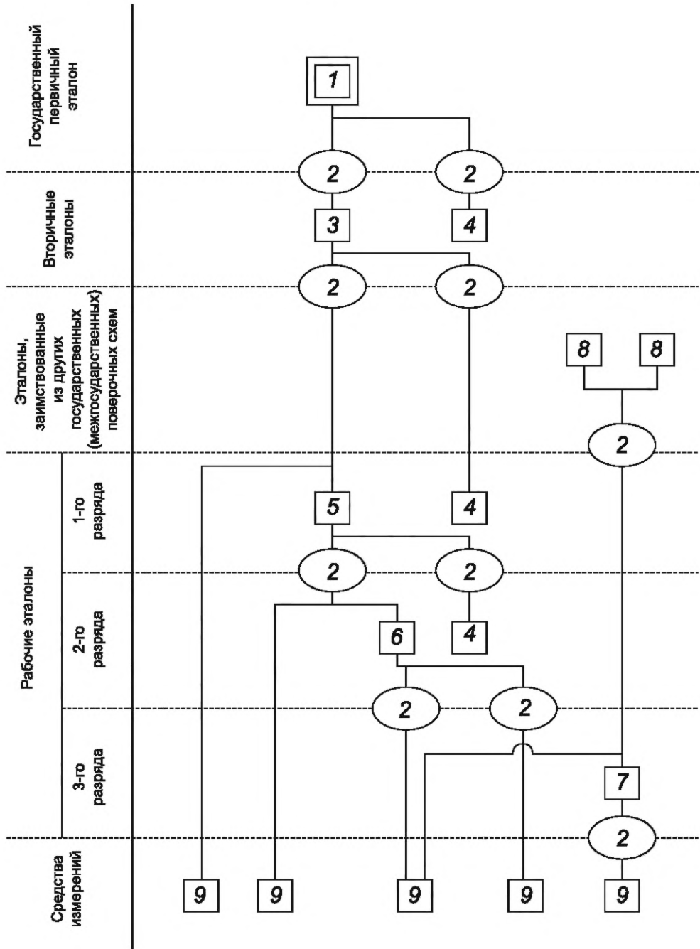
Пример компоновки государственной поверочной схемы
