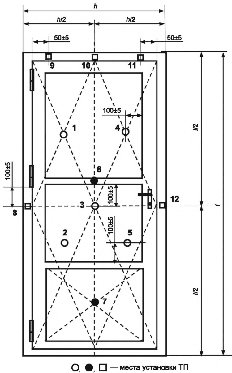
Рисунок В.5 — Схема установки ТП на необогреваемой поверхности однопольного дверного блока
