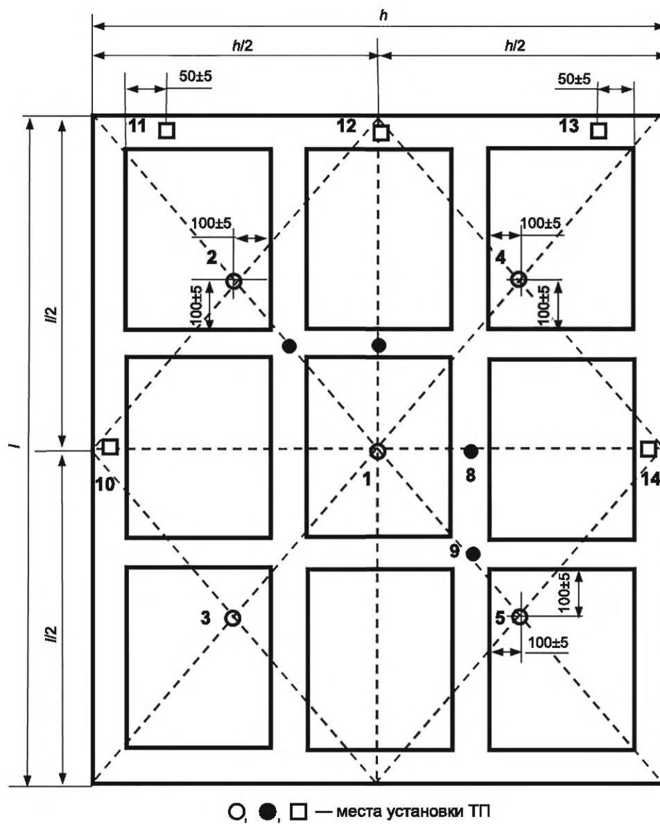
Рисунок В.2 — Схема установки ТП на необогреваемой поверхности перегородки
