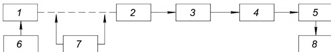
1, 2, 4 — развязывающие устройства; 3 — измерительный аттенюатор; 5 — детекторная головка; 6 — генератор сигналов ВЧ и СВЧ; 7 — изделие; 8 — индикатор
