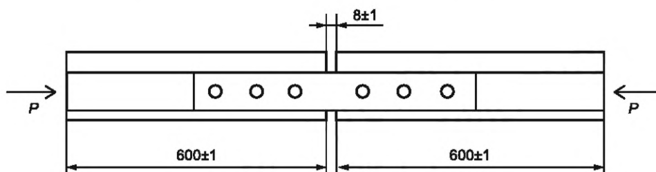
б) Схема испытаний по оценке продольной несущей способности при сжатии
