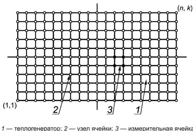
Рисунок 3 — Измерительная сетка
