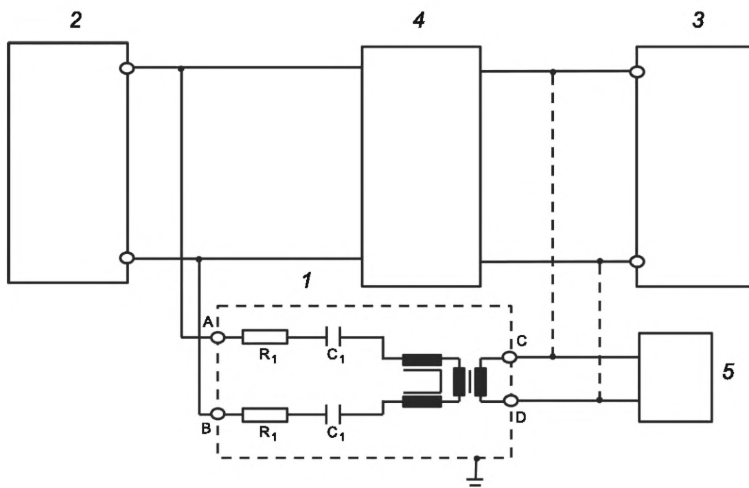
1 — AAN; 2 — транспортное средство; 3 — зарядная станция/источник питания; 4 — HV-AN или AMN или DC-charging-AN; 5 — AE; A — PLC по линии питания переменного или постоянного тока (на стороне транспортного средства); B — PLC по линии питания переменного или постоянного тока (на стороне транспортного средства); C — линия PLC (на стороне зарядной станции или AE); D — линия PLC (на стороне зарядной станции или AE); R_1 — 2,5 кОм; C_1 — 4,7 мкФ
