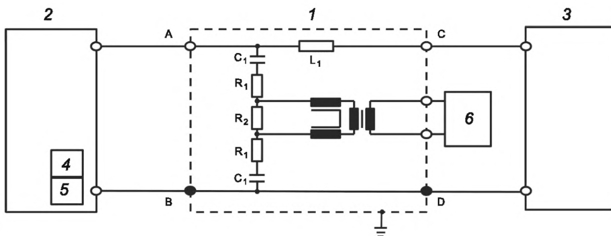
1 — AAN; 2 — транспортное средство; 3 — зарядная станция; 4 — блок сигналов управления (в транспортном средстве); 5 — PLC (в транспортном средстве); 6 — AE; A — контрольная линия управления (со стороны транспортного средства); B/D — защитное заземление; C — контрольная линия управления (со стороны зарядной станции); R_1 — 39 Ом; R_2 — 270 Ом; C_1 — 2,2 нФ; L_1 — 100 мкГн
