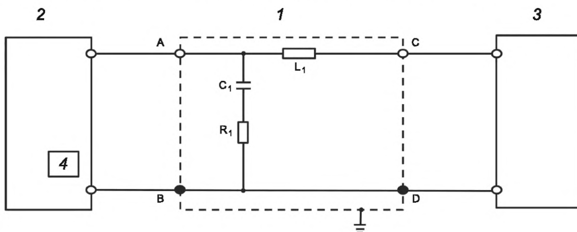
1 — AAN; 2 — транспортное средство; 3 — зарядная станция; 4 — блок сигналов управления (в транспортном средстве); A — линия управления (со стороны транспортного средства); B/D — защитное заземление; C — контрольная линия управления (со стороны зарядной станции); R_1 — 150 Ом; C_1 — 1,1 нФ; L_1 — 100 мкГн
