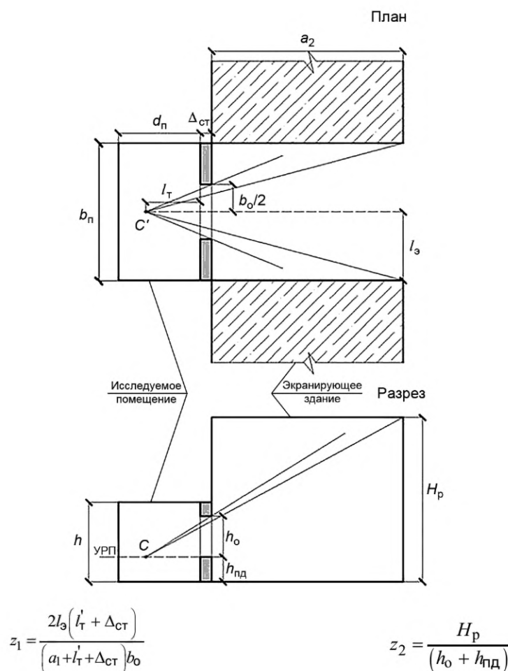
Рисунок А.4 — Схема № 4 к определению параметров П-образной застройки с расчетным зданием, расположенным между двух параллельных зданий
