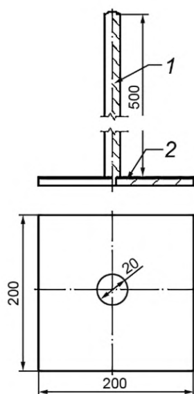
Рисунок Б.1 — Конструкция грунтовой деформационной марки
