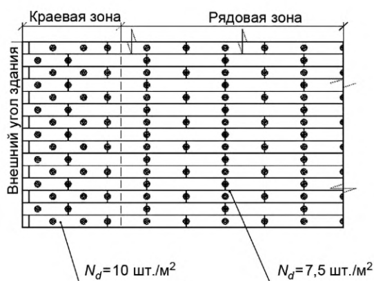
Пример фрагмента теплоизоляции стен выше отм. +40,0 от уровня отмостки здания
