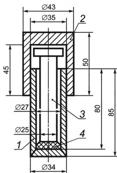
Рисунок Б.3 — Конструкция и размеры стаканчика
