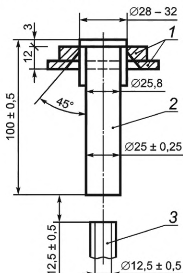
Рисунок Б.2 — Установка для закалки образца
