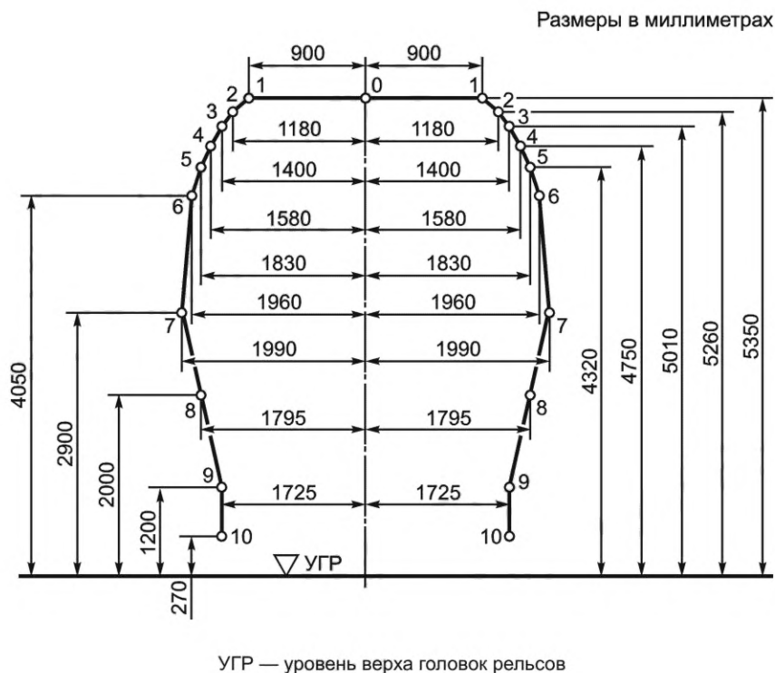
Рисунок А.2 — Контрольное очертание сооружений Ц для пропуска подвижного состава габарита T_c при скорости движения более 40 км/ч
