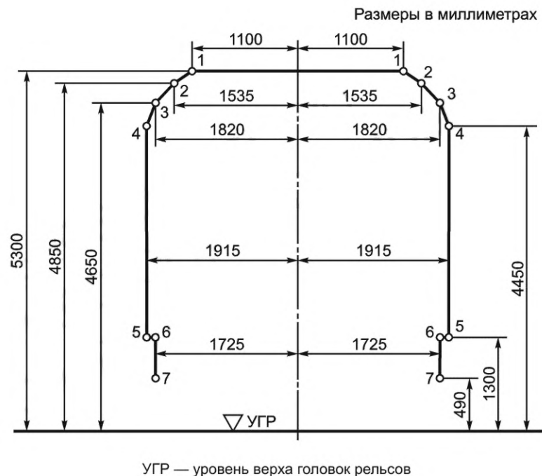
Рисунок А.1 — Контрольные очертания приближения строений КО для пропуска пассажирских вагонов и полувагонов габарита T_{пр}
