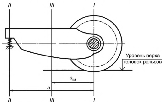
Рисунок И.1 — Схема полуобрессоренной детали
