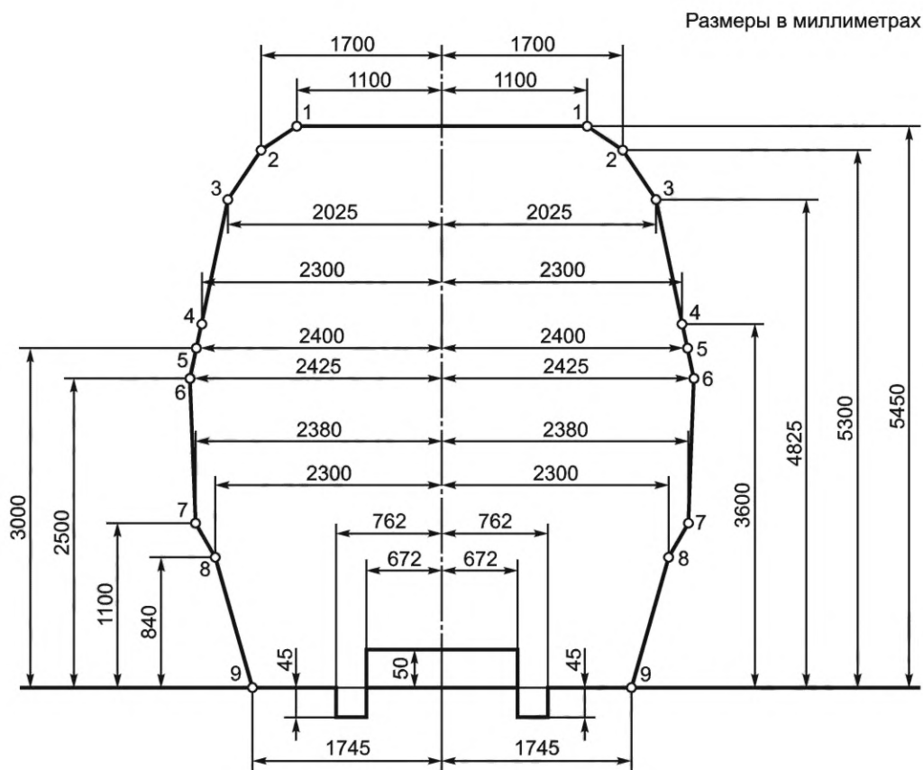
Рисунок Д.3 — Минимальное внутреннее очертание переустриваемых существующих сооружений (для не электрифицированных линий)
