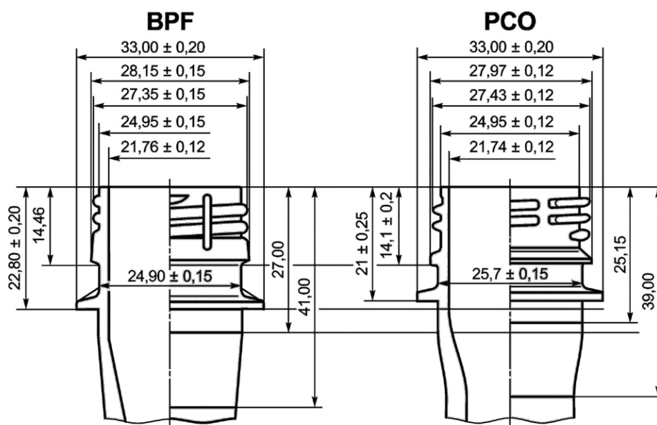
Рисунок Б.1 — Типы преформ
