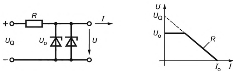
b) — Трапецевидные характеристики
