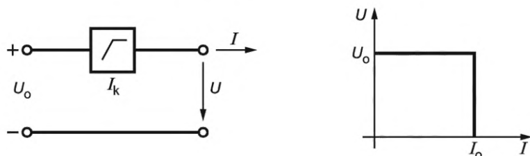
с) — Прямоугольные характеристики
