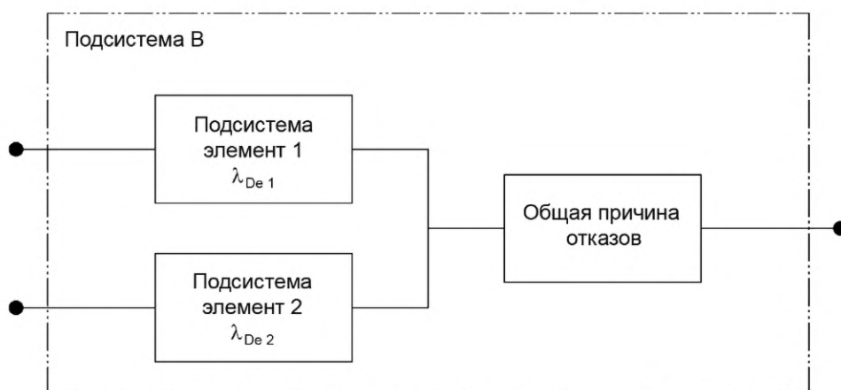
Рисунок К.4 — Логическое представление базовой архитектуры подсистемы типа В
