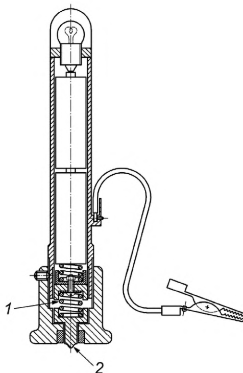
1 — пружина с усилием нажатия 10 Н; 2 — наконечник, которым производится царапание (стальной шарик диаметром 1 мм)
