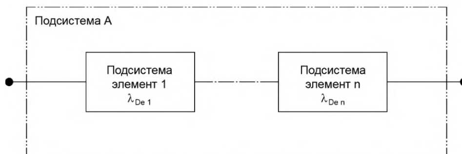
Рисунок J.1 — Логическое представление базовой архитектуры подсистемы типа A
