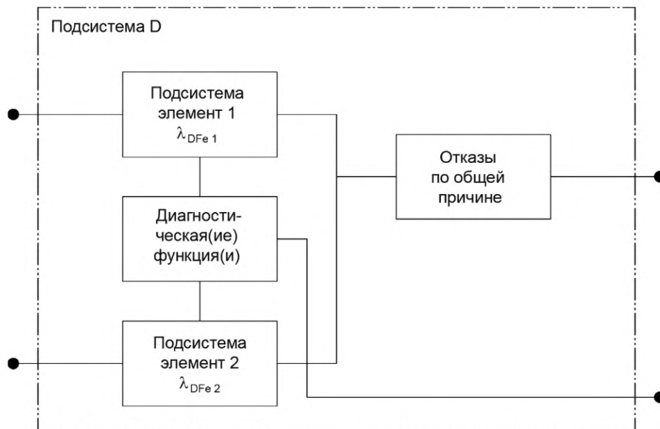
Рисунок J.4 — Логическое представление базовой архитектуры подсистемы типа D
