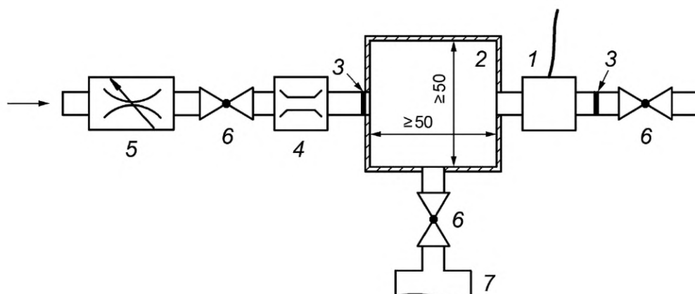
1 — испытуемый образец; 2 — испытательная камера; 3 — огнегасительное устройство; 4 — расходомер; 5 — ограничитель; 6 — клапан; 7 — разрывная мембрана
