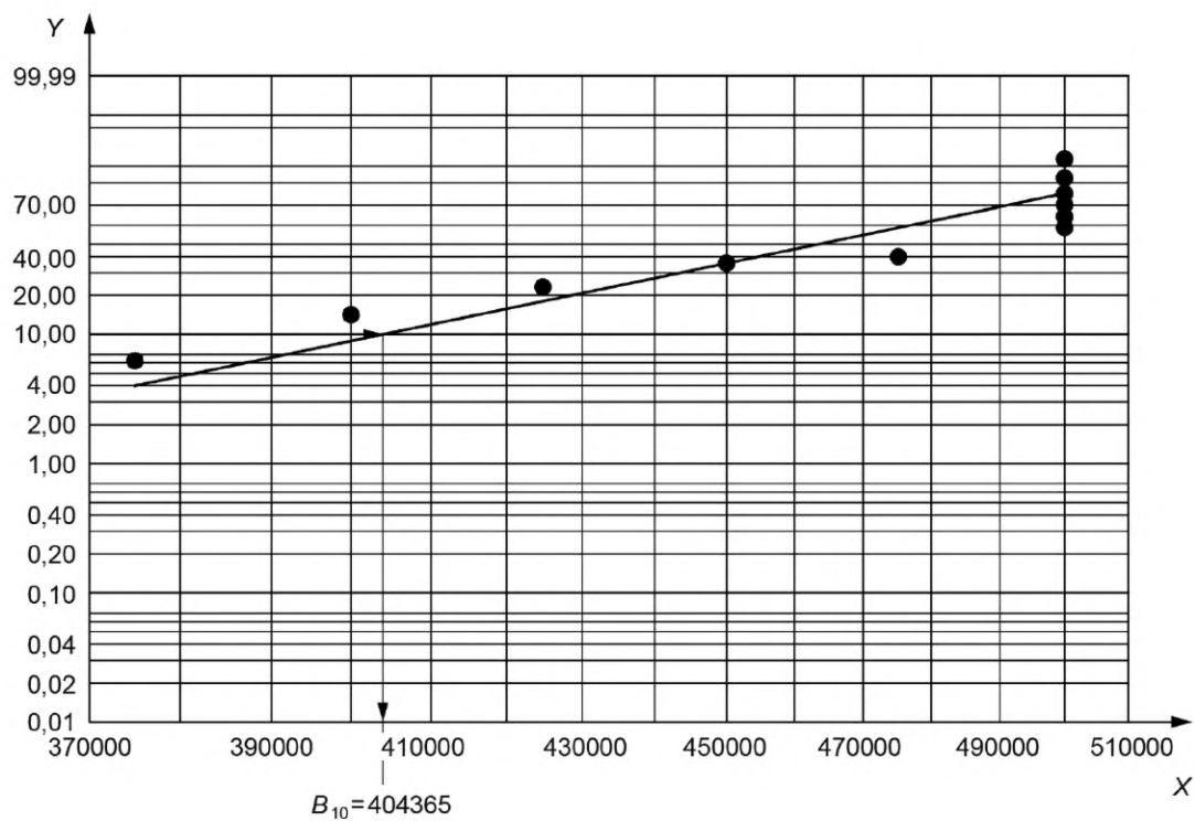
Рисунок К.2 — Пример А распределения Вейбулла (максимальная длительность испытания составляет 500 000 циклов)
