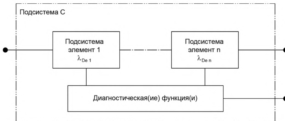
Рисунок J.2 — Логическое представление базовой архитектуры подсистемы типа С
