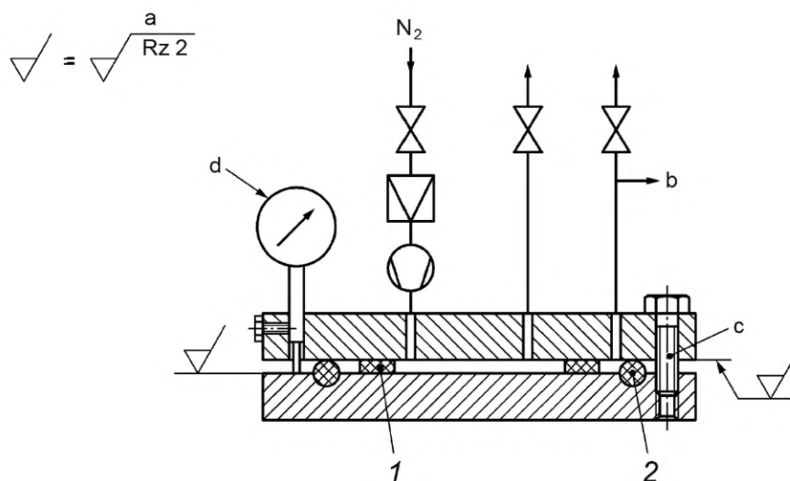
1 — уплотнение; 2 — О-кольцо; Rz — шероховатость; а — полированная; b — газовая бюретка для газа; с — 6 болтов по периметру; d — 3 микрометра
