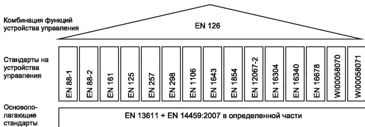
Рисунок 1 — Взаимосвязь стандартов на устройства управления
