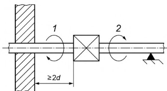
Рисунок 5 — Схема испытания крутящим моментом
