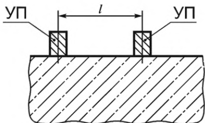
б — схема испытания бетона при поверхностном прозвучивании
