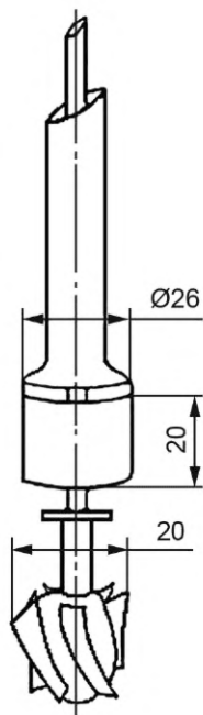
Рисунок 2 — Винтовая мешалка
