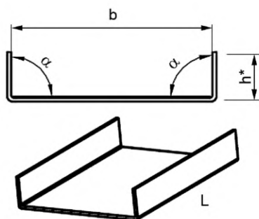
Рисунок А.6 — Элемент обрамления
