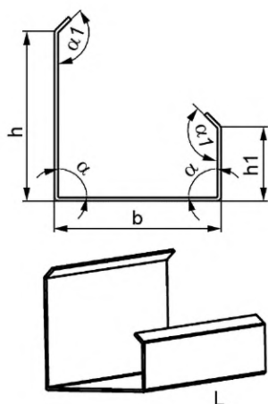
Рисунок А.7 — Элемент жесткости
