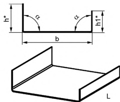
Рисунок А.5 — Элемент усиления
