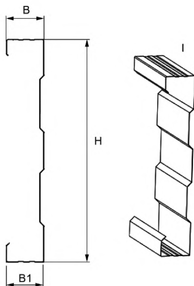
Рисунок А.1 — Начальный сэндвич-профиль
