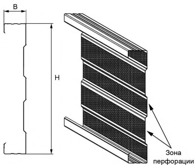
Рисунок А.3 — Начальный акустический сэндвич-профиль
