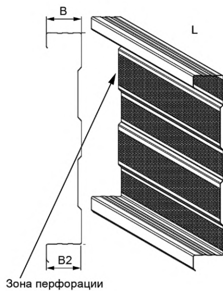
Рисунок А.4 — Рядовой акустический сэндвич-профиль
