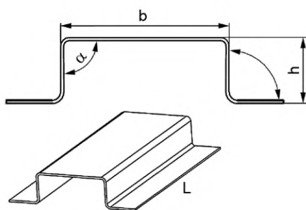
Рисунок А.10 — Шляпный крепежный профиль
