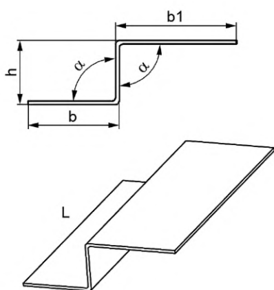
Рисунок А.9 — Z-образный крепежный профиль
