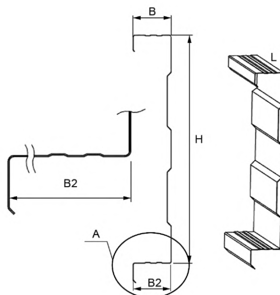
Рисунок А.2 — Рядовой сэндвич-профиль
