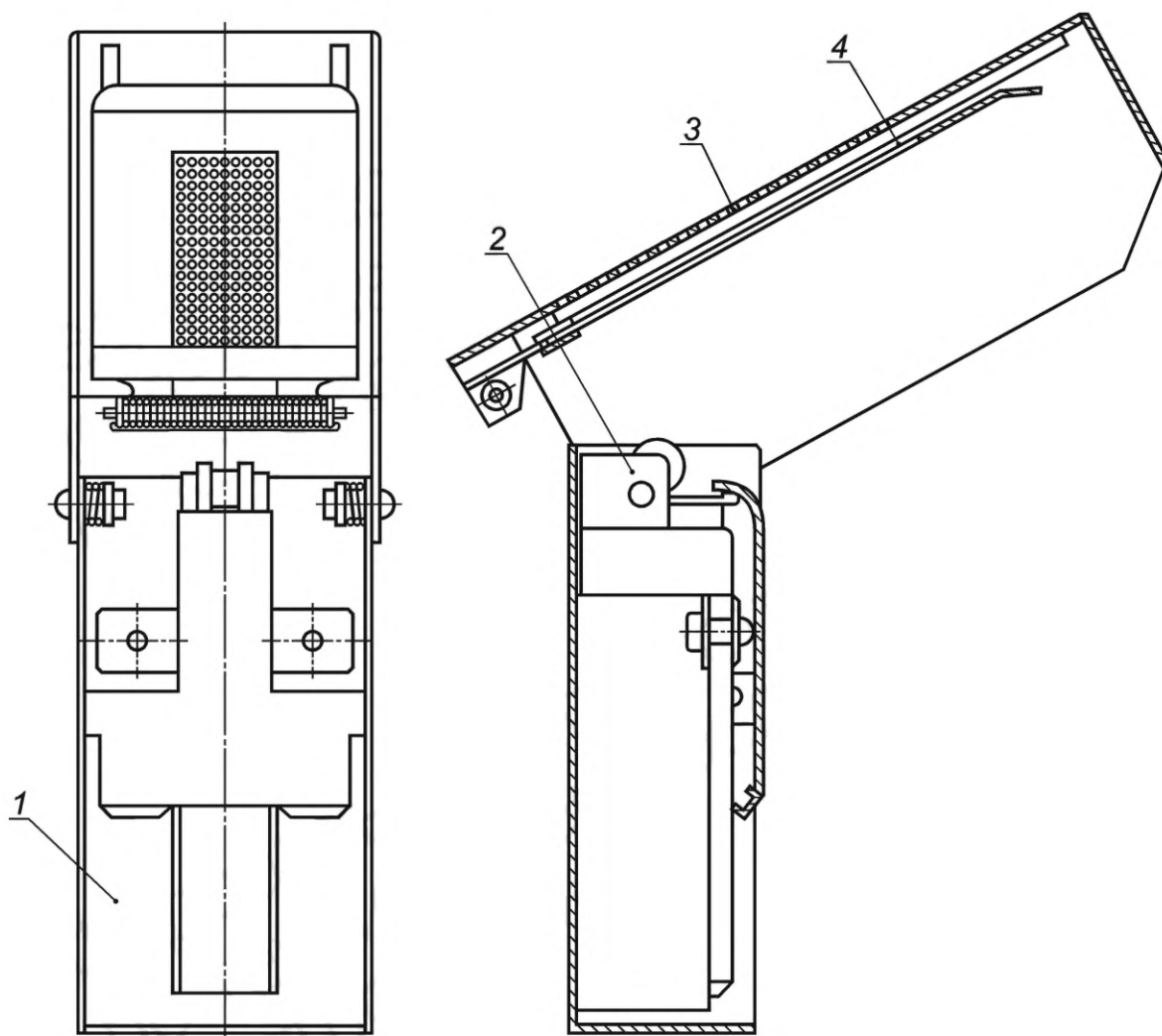
1 — корпус; 2 — газовая зажигалка; 3 — поворотная крышка; 4 — зажимное устройство
