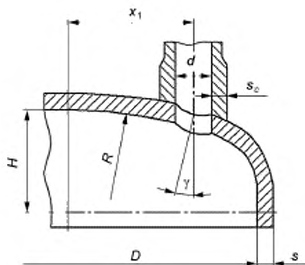
Рисунок 6.6 — Смещенный штуцер на эллиптическом днище
